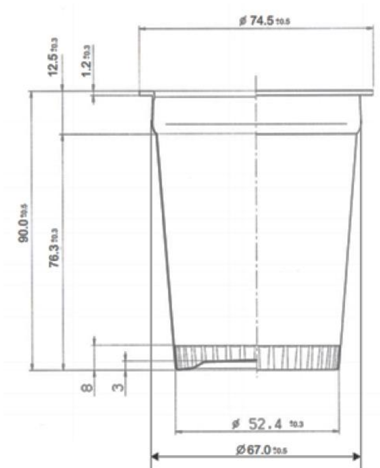
Figura 1 – Unidade dimensional do copo em milímetro (75mmx90mm)
